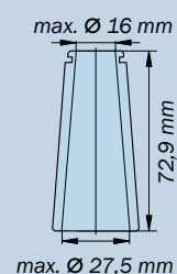
Hűtőelem adapterrel a hosszabbítóval felszerelt zsugortokmányhoz Cooling body with adapter for shrink
