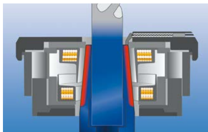
Nagyméretű szerszám/Big tool
