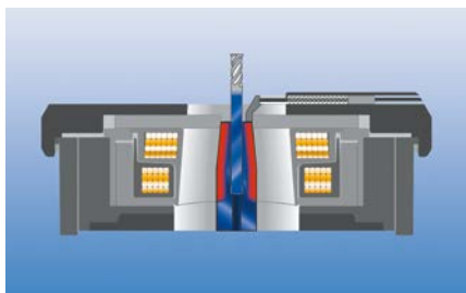
Kisméretű szerszám/Small tool
