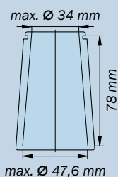
Hűtőelem adapterrel speciális zsugortokmányokhoz Cooling body with adapter for special shrink fit chucks
